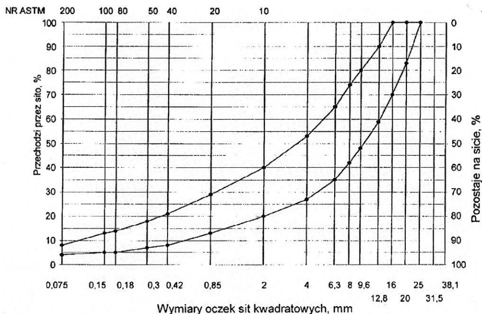
Rys. 1. Krzywe graniczne uziarnienia mieszanki mineralnej BA od 0 do 20 mm do podbudowy nawierzchni drogi o obciążeniu ruchem KR 2
