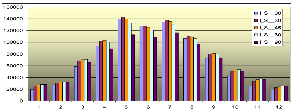
Rysunek 21. Średnia miesięczna energia promieniowania słonecznego (Wh/m 2 ) dla stacji meteorologicznej Toruń w zależności od miesiąca i kąta nachylenia dla kierunku południowego
